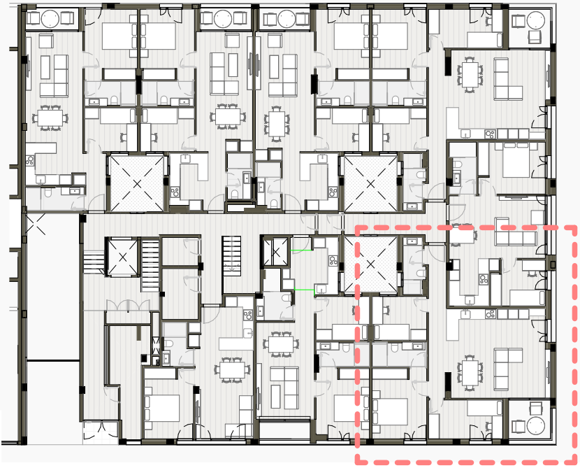
PLANTA BAJA
